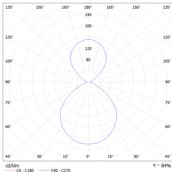
diagramma polare
