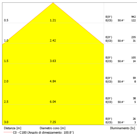
Diagramma conico
